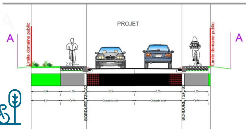
Aménagement d'une piste cyclable entre Cuverville et Démouville
